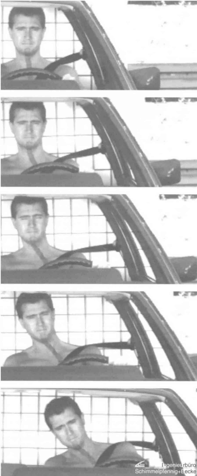
Bild 2 Bewegungsablauf eines Insassen auf der stoßabgewandten Seite, \Delta v = 8,0 \text{ km/h} Fig. 2 Motion of occupant from impact, Delta-V 8,0 km/h
