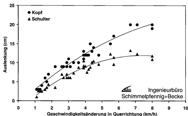
Bild 4 Abhängigkeit der seitlichen Kopf- und Schulterausslenkung von der Geschwindigkeitsänderung in Querrichtung
