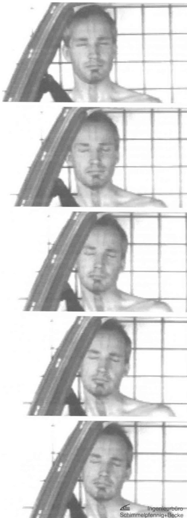
Bild 5 Bewegungsablauf eines Insassen auf der stoßzugewandten Seite, \Delta v = 5,1 km/h Fig. 1 Motion of occupant toward impact, Delta-V 5,1 km/h
