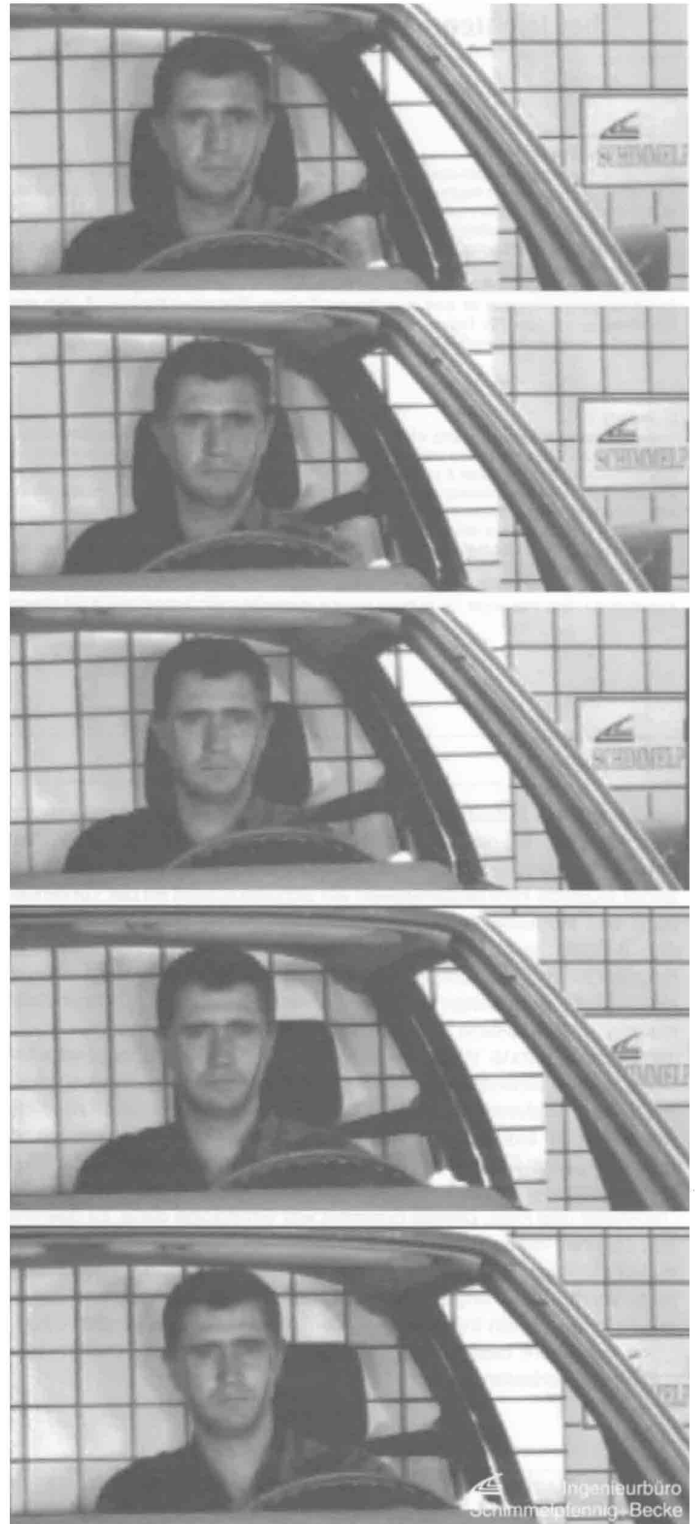
Bild 3 Bewegungsablauf eines Insassen auf der stoßzugewandten Seite, \Delta v = 3,0 \text{ km/h} Fig. 3 Motion of occupant away from impact, Delta-V 3,0 km/h
