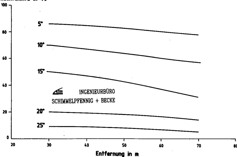
Bild 1 Prismenöffnung abgewandt
